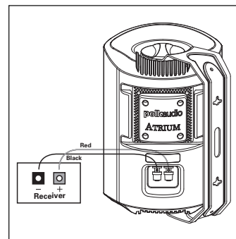
FIGURE 16: Connecter le fil de haut parleur aux bornes.
