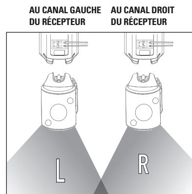
PAIRE D'ENCEINTES STÉRÉO (ENTRÉE SIMPLE)
